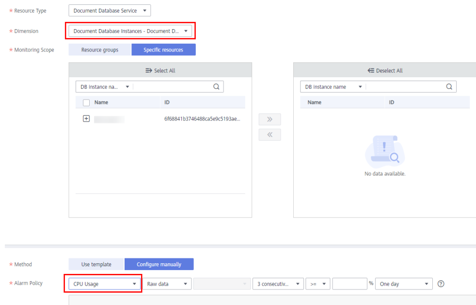
Figura 16-1 Configuración de la dimensión de monitoreo
